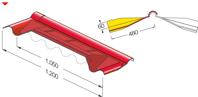
Zweiteilige Firsthaube, variable Neigung aus Polimglass® für Onda 177
