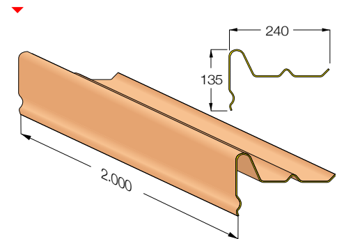
Ortgangwinkel aus Polimglass®
